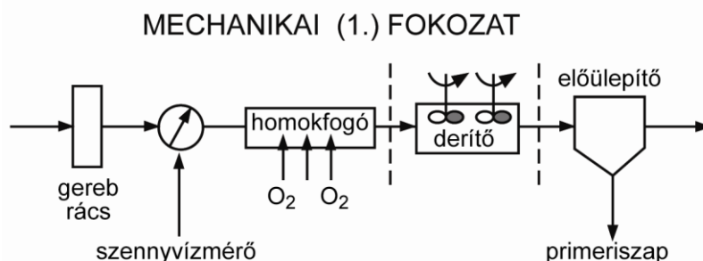
6.6.1. ábra: A háromfokozatú, eleveniszapos szennyvíztisztítási technológia mechanikai fokozatának folyamatábrája
