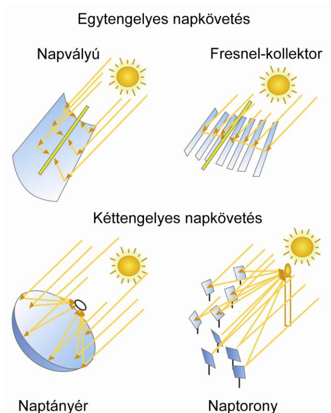
3.12.4. ábra: Termovillamos naperőművek vázlatos áttekintése (Forrás: WEC 2007. alapján)
