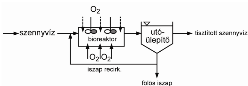
6.6.3. ábra: A háromfokozatú, eleveniszapos szennyvíztisztítási technológia biológiai fokozatának folyamatábrája
