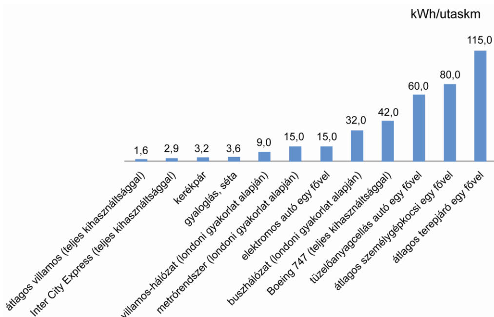
3.9.1. ábra: Különbözo közlekedési módok energiahatékonysága (MacKay, D. 2009 alapján)
