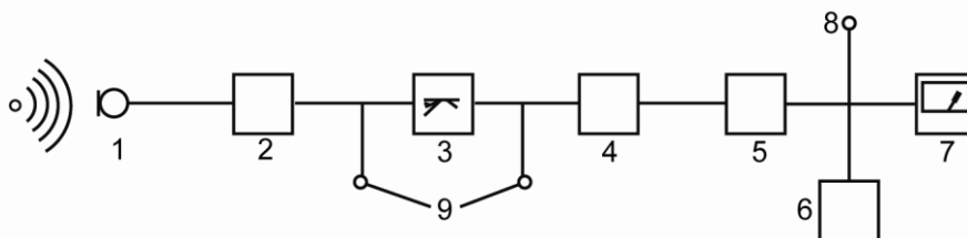
8.4.1. ábra: A hangszintmérő vázlatos felépítése (Forrás: Moser–Pálmay: A környezetvédelem alapjai Bp. 1999. p. 385.)
