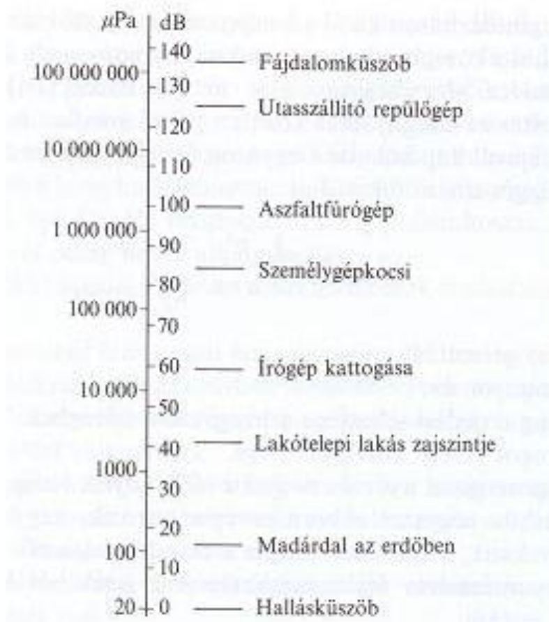
8.1.1. ábra: Az egyes hangforrások hangnyomásértékei (Pa), illetve hangnyomásszintjei (dB) (Forrás: Moser–Pálmai: A környezetvédelem alapjai Bp., 1999., pp. 364.)
