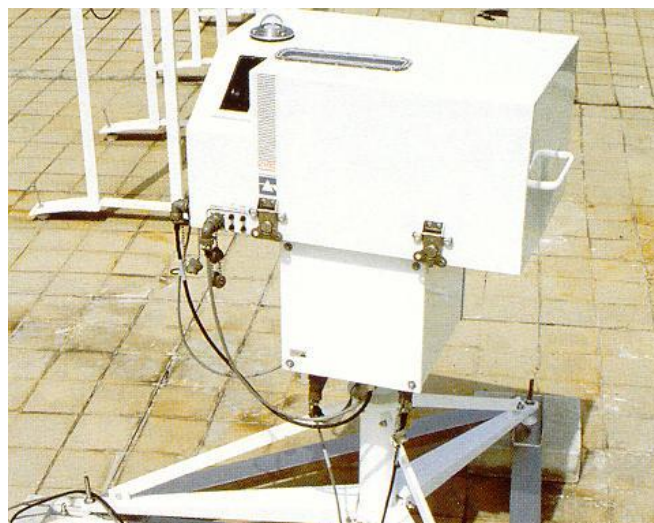
7.4.6. ábra: Brewer-féle spektrofotométer (Forrás: OMSz)
