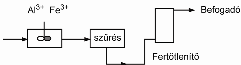
6.6.5. ábra: A háromfokozatú, eleveniszapos szennyvíztisztítási technológia terciér fokozatának folyamatábrája
