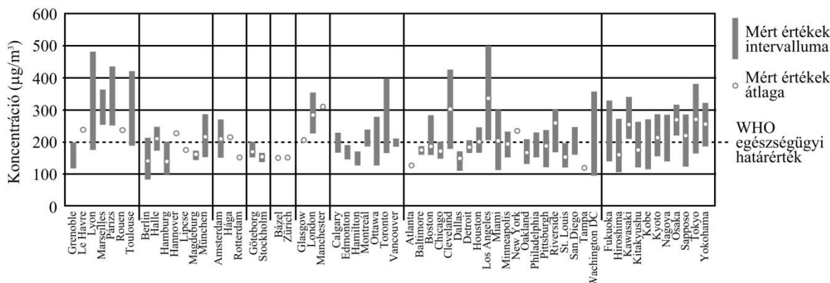
7.2.11. ábra: A városi csúcsgorgalom idején mért óras NO 2 -szint (Forrás: OECD/ENV, 1998)
