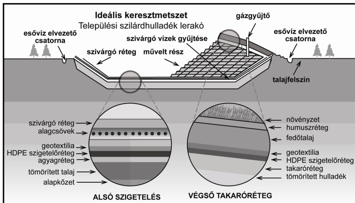
4.5.9. ábra: Egy ideális települési szilárdhulladék-lerakó alsó és felső rétegrendje (Forrás: Szilágyi L., 2010)
