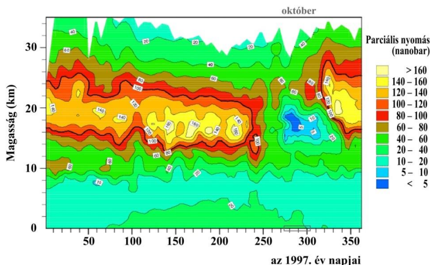
7.4.17. ábra: Az ózon parciális nyomásának vertikális eloszlása 1997 során rádiószondás mérési adatok alapján, Neumayer ( 70^{\circ}39' \text{ D} , 8^{\circ}15' \text{ Ny} ) (Forrás: NASA)
