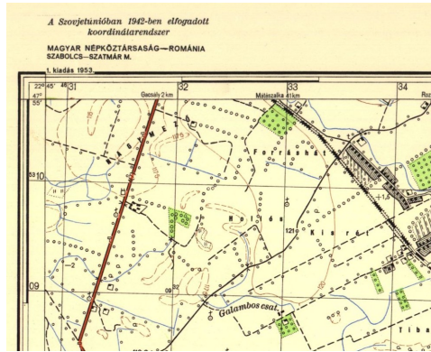
26. ábra. A Gauss-Krüger térképek szelvényhatárai a szélességi és hosszúsági köröket követik.
