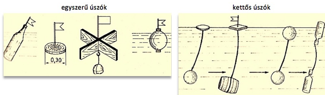
5.7. ábra. A vízsebességmérő úszók típusai (forrás: Boros L. 1985. 269–270. o.)
