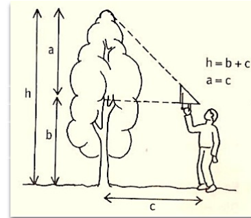
2.15. ábra. Tereptárgy magasságának becslése háromszögvonalzóval
