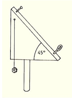
2.15. ábra. Tereptárgy magasságának becslése háromszögvonalzóval
